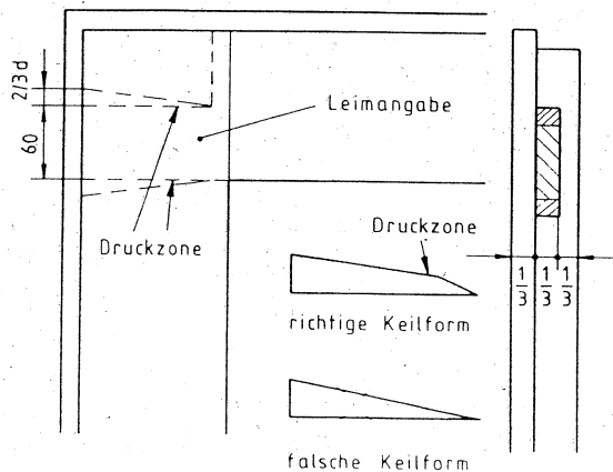
Gestemmte Rahmenecke
