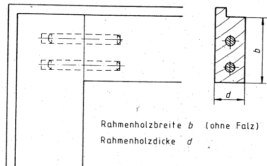
Gedübelte Rahmenecke
