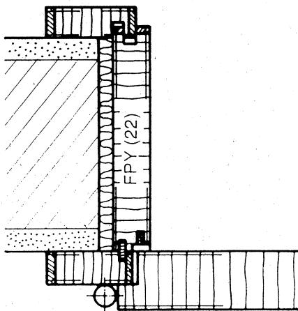
Konstruktion mit Futter und Bekleidungen, schwere Tür mit Doppeldichtung
