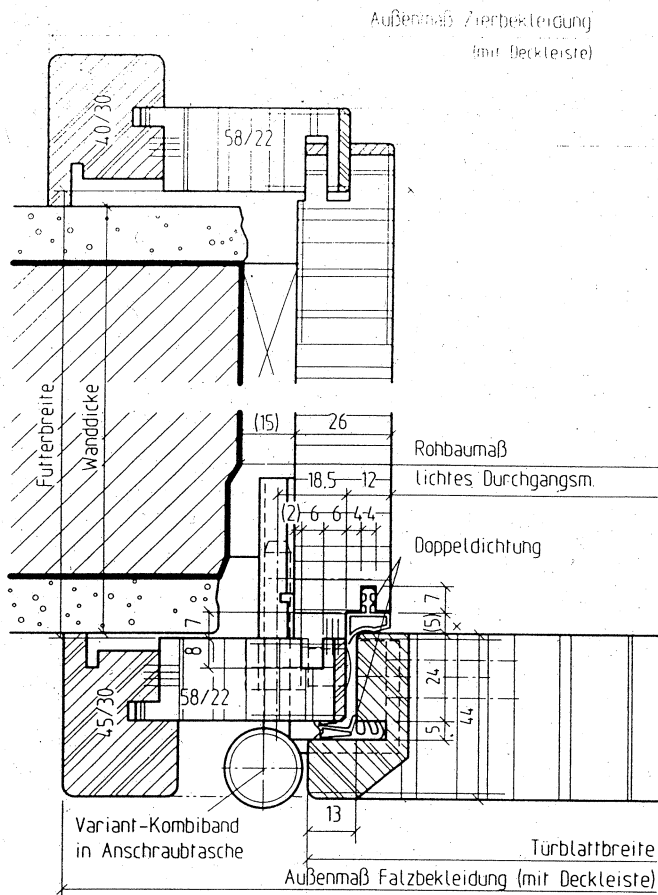
Konstruktion mit Futter und Bekleidungen, schwere Tür mit Doppeldichtung
