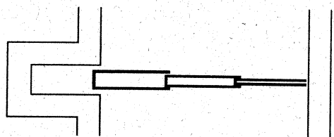
Teleskoptüre
